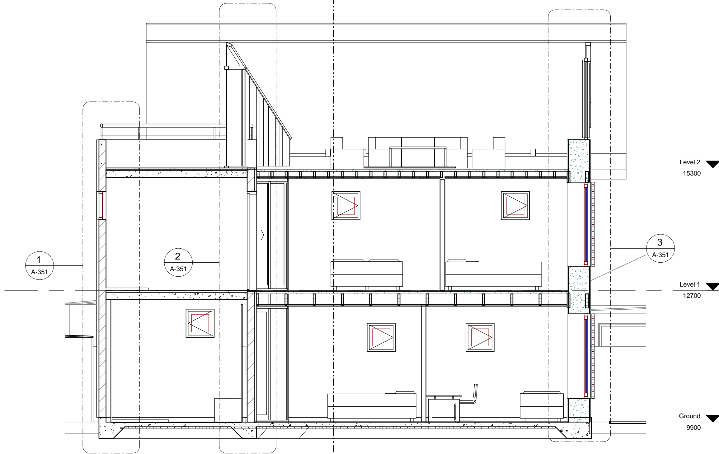
2 Section 2 A100 1 : 50
