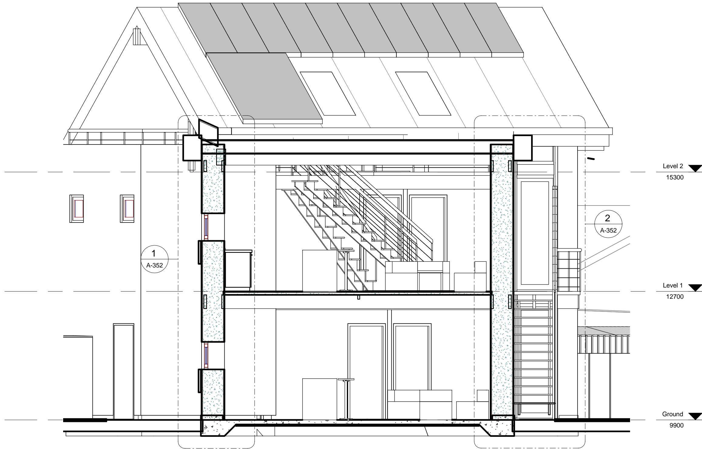
1 Section 3 A100 1 : 50
